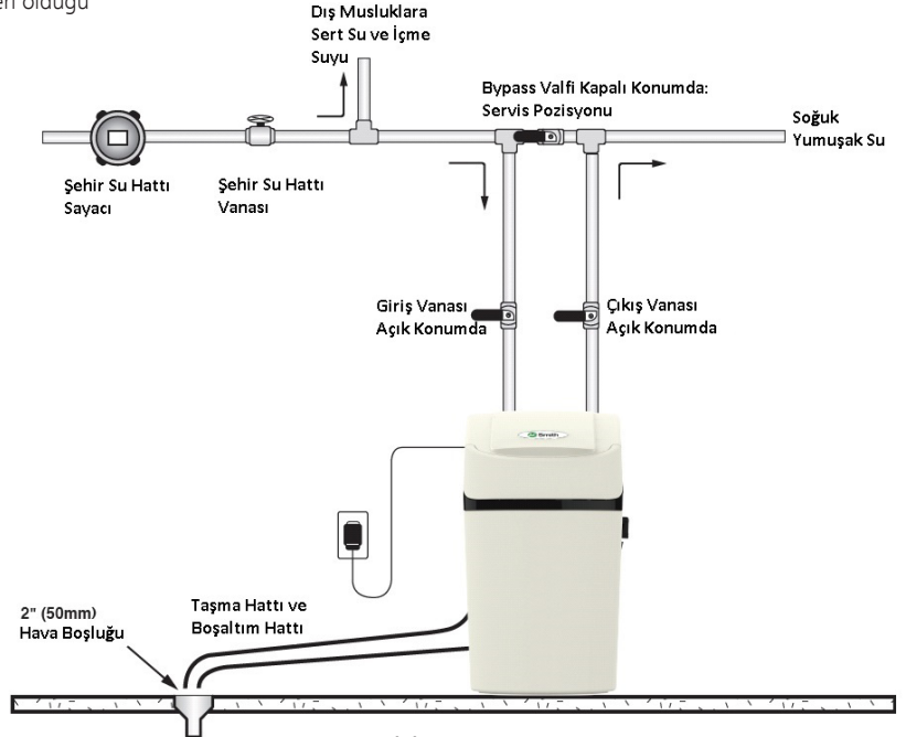
Şekil 12: Bypass Pozisyonu
