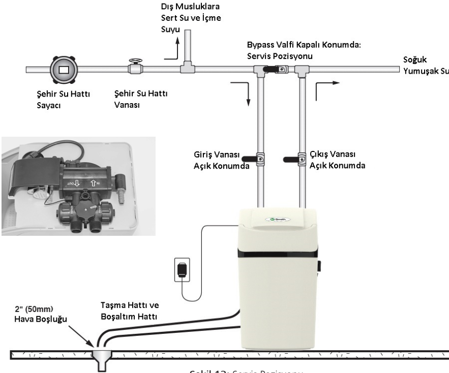
Şekil 13: Servis Pozisyonu
