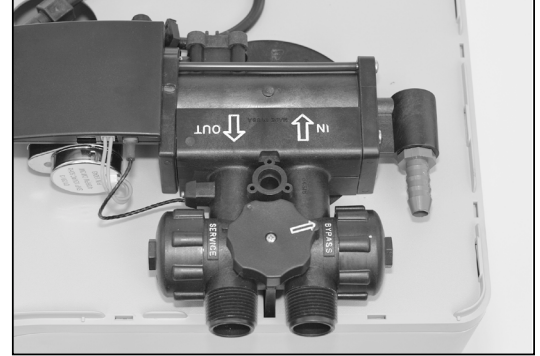
Şekil 17: Bypass Valfi
