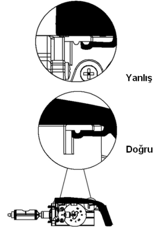
Şekil 14: Kontrol Cihazı Sekme Kilit Ayırntısı
